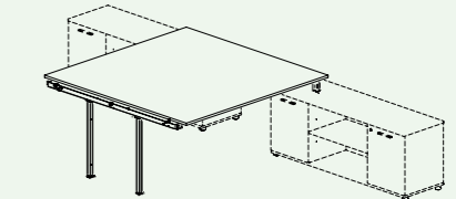
POSTAZIONE AGGIUNTIVA Additional workstation | Poste de travail supplémentaire
