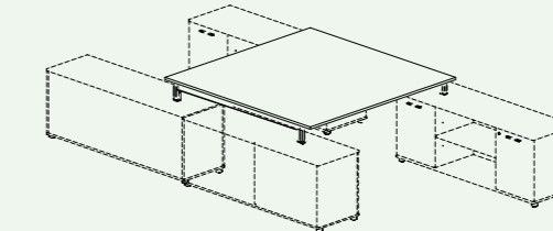
POSTAZIONE CONDIVISA CON CONTENITORE DI SUPPORTO Shared workstation with support container | Poste de travail partagé avec conteneur de support
